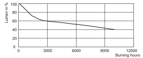
CDM-R111 35W /942
