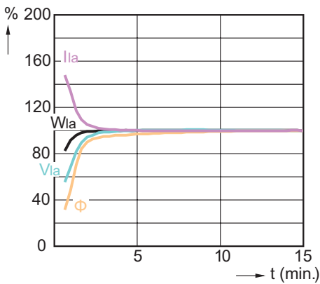
CDM-R111 35W /942
