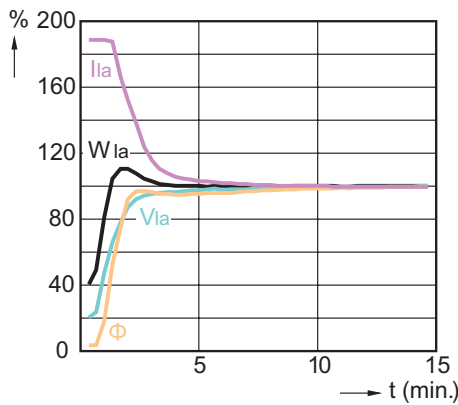
CDM-R111 70W /942
