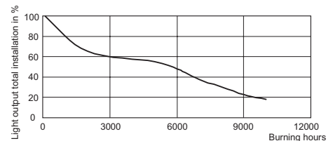
CDM-R111 35W /942
